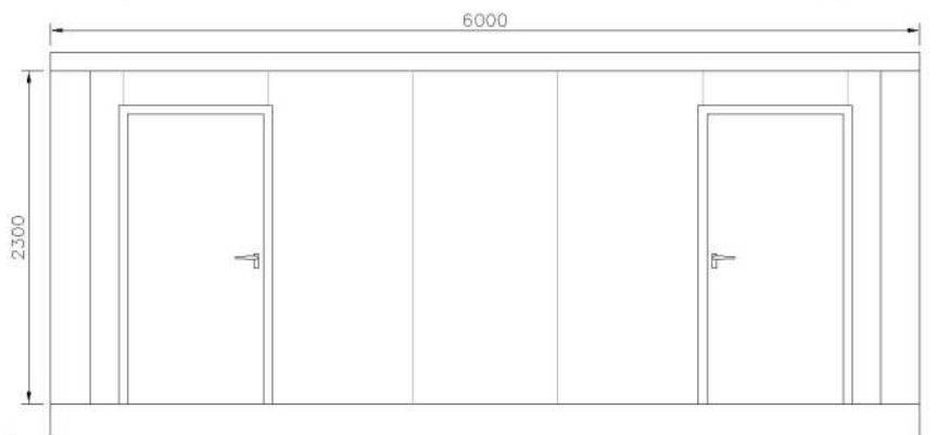
Alçado principal
