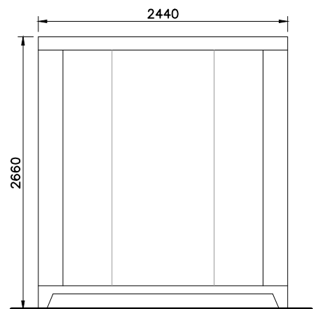
Alçado lateral direito
