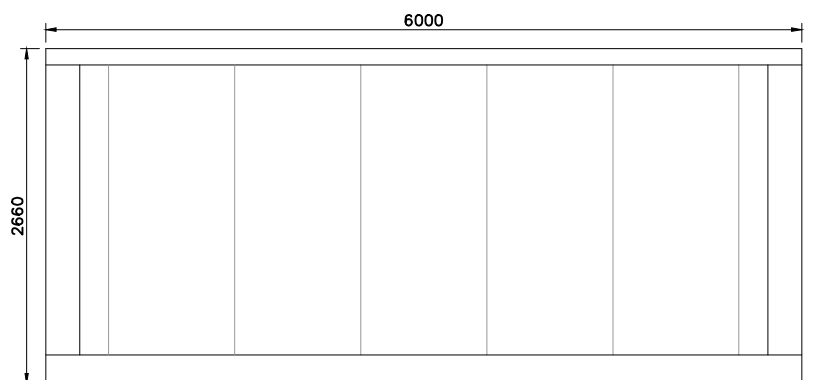
Alçado posterior
