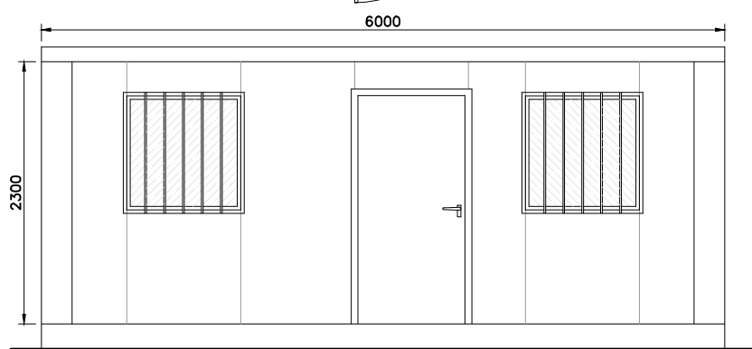
Alçado principal
