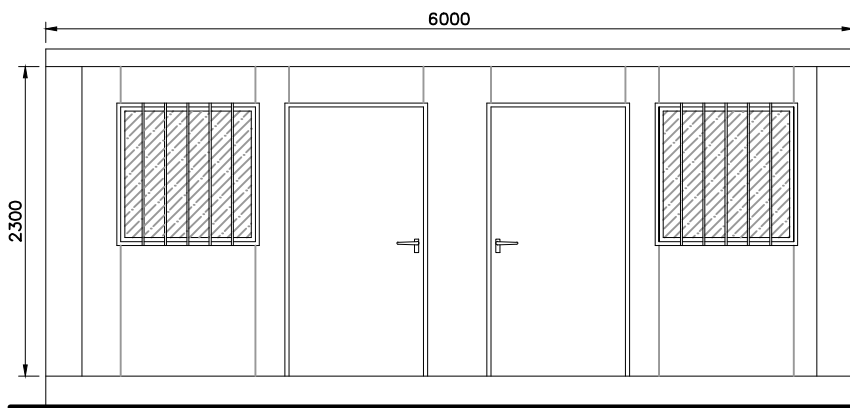
Alçado principal
