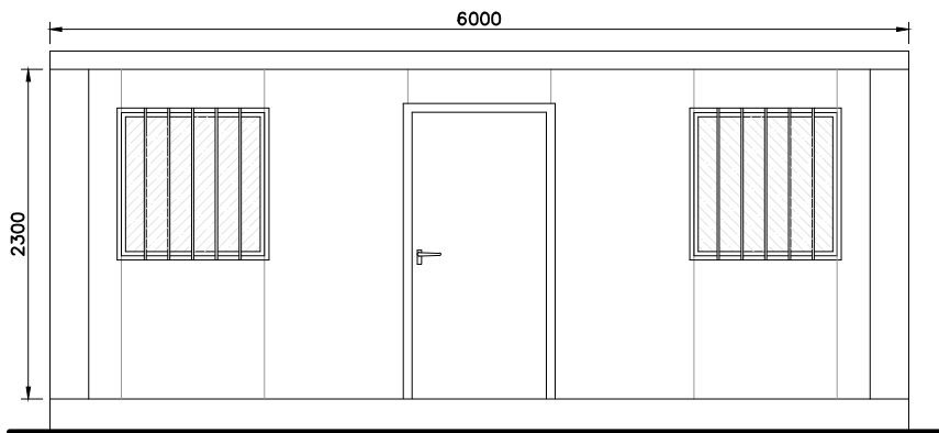
Alçado principal
