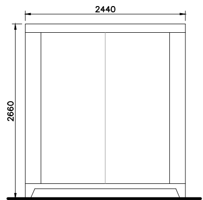
Alçado lateral
