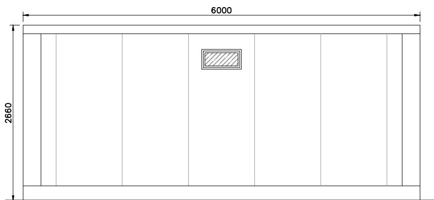
Alçado posterior
