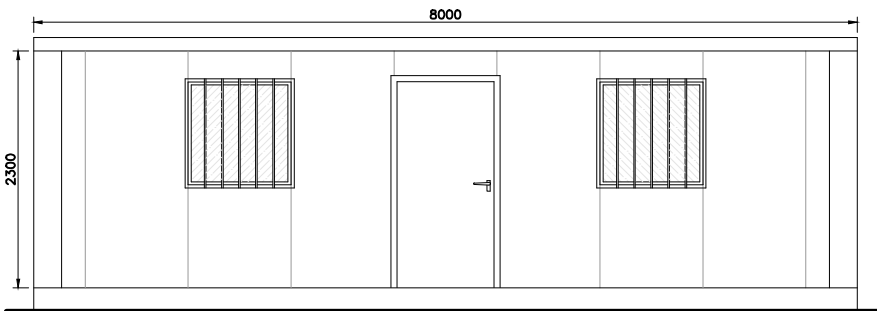
Alçado principal
