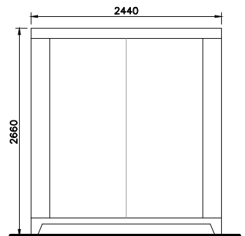
Alçado lateral
