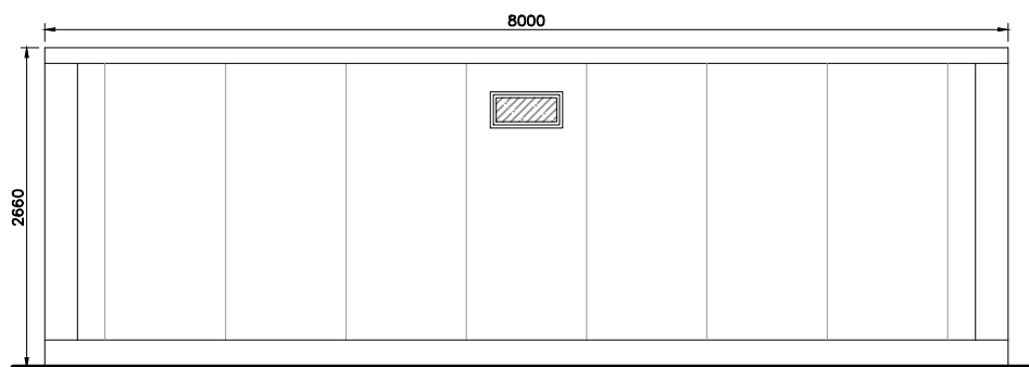
Alçado posterior
