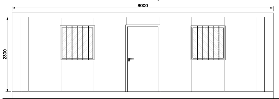
Alçado principal
