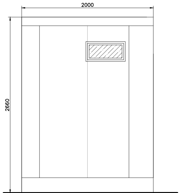
Alçado lateral esquerdo
