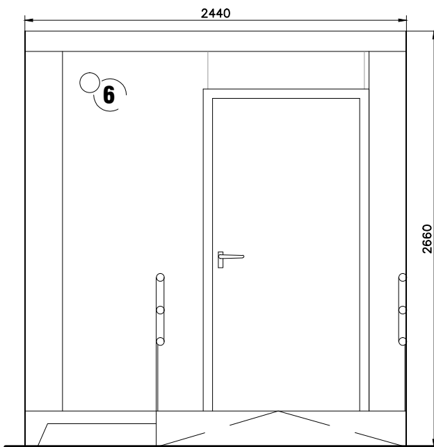
Alçado Principal
