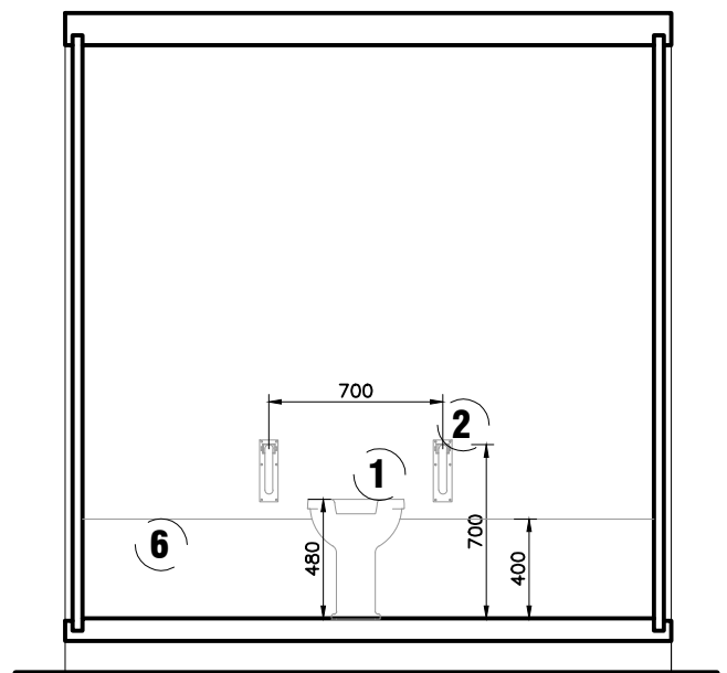
Corte AA'
