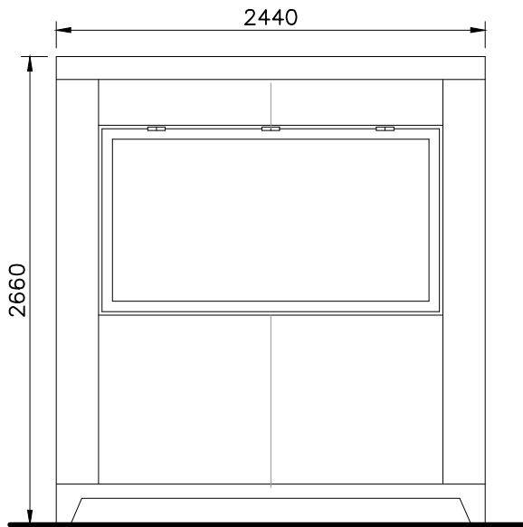
Alçado principal
