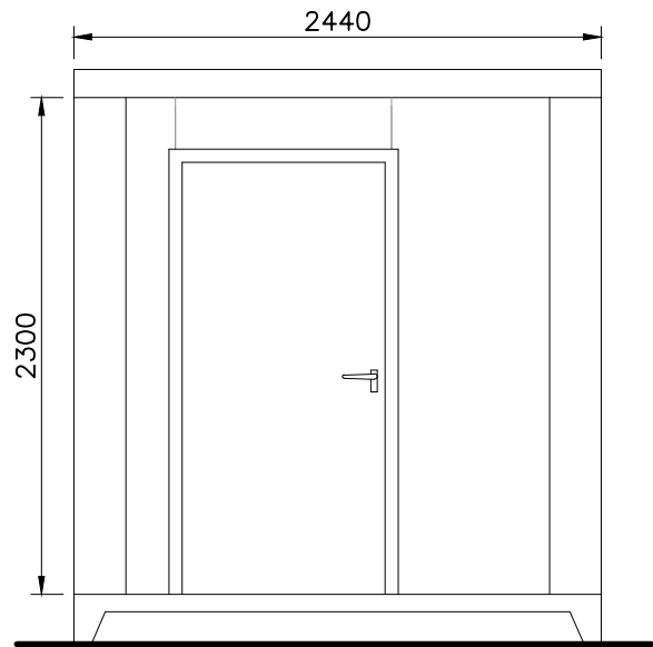
Alçado posterior
