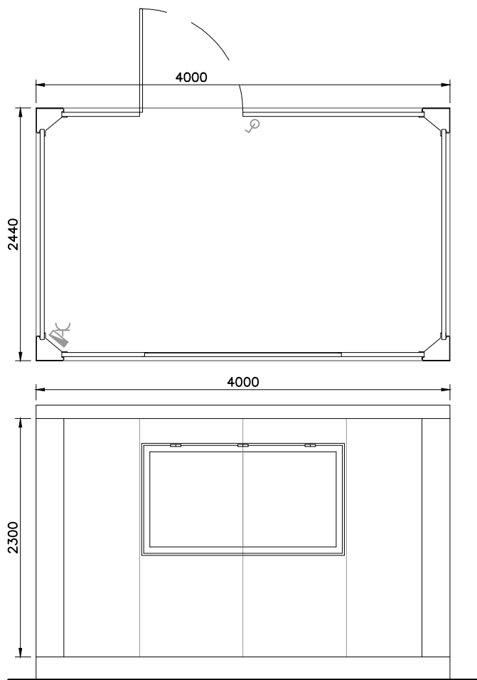
Alçado principal
