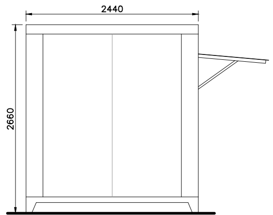
Alçado lateral
