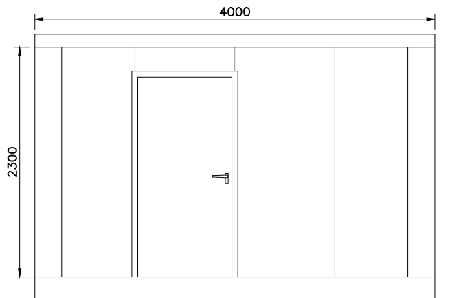
Alçado principal
