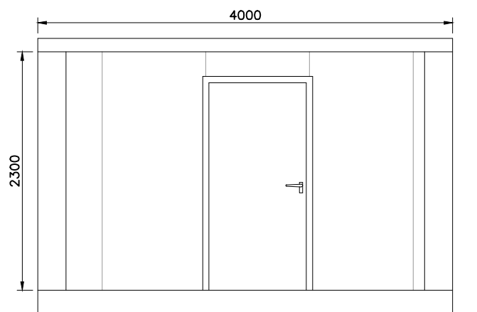
Alçado principal
