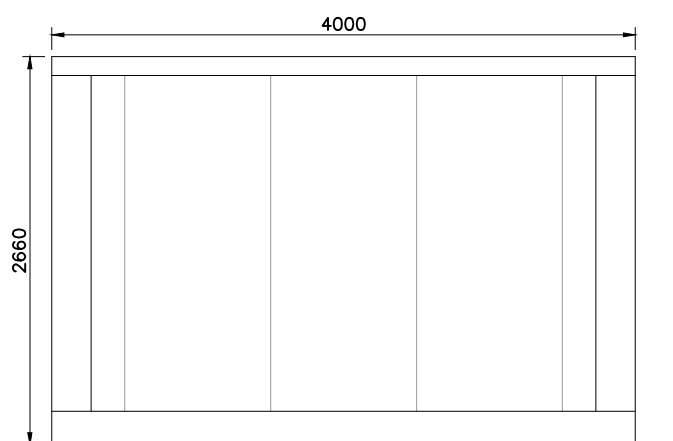
Alçado posterior
