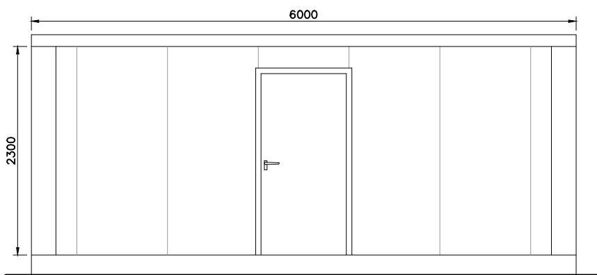
Alçado principal
